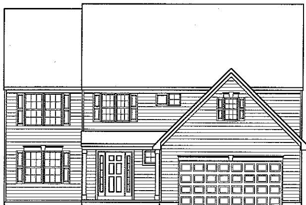
ELEVATION A-10
