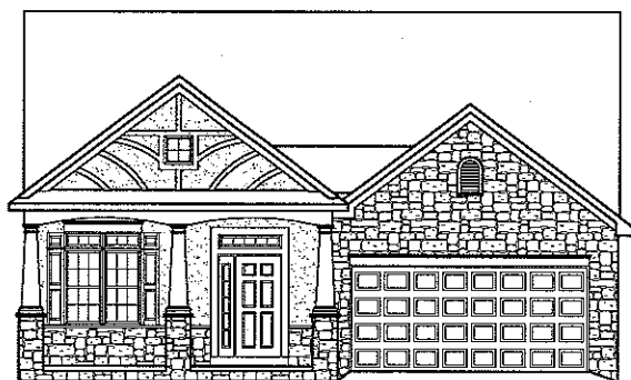
ELEVATION C-20
