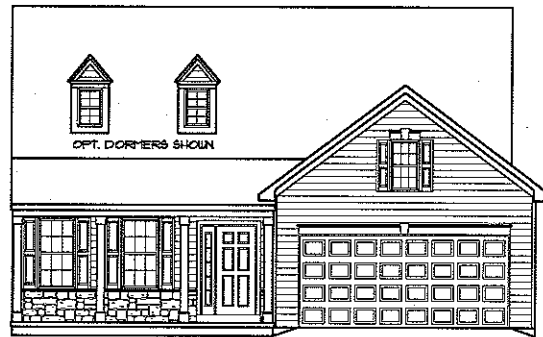
ELEVATION A-20
