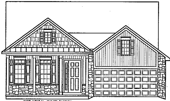
ELEVATION B-10
