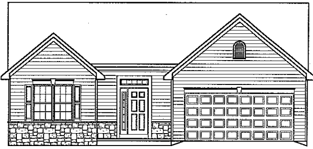
ELEVATION A-10
