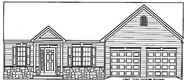
ELEVATION A-20
